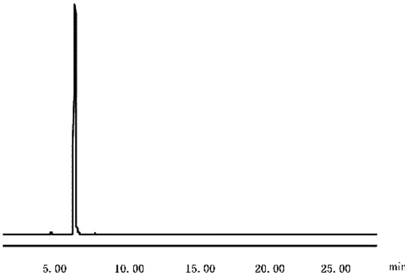
图 B.1 甲醛-2,4-二硝基苯腙参考色谱图
