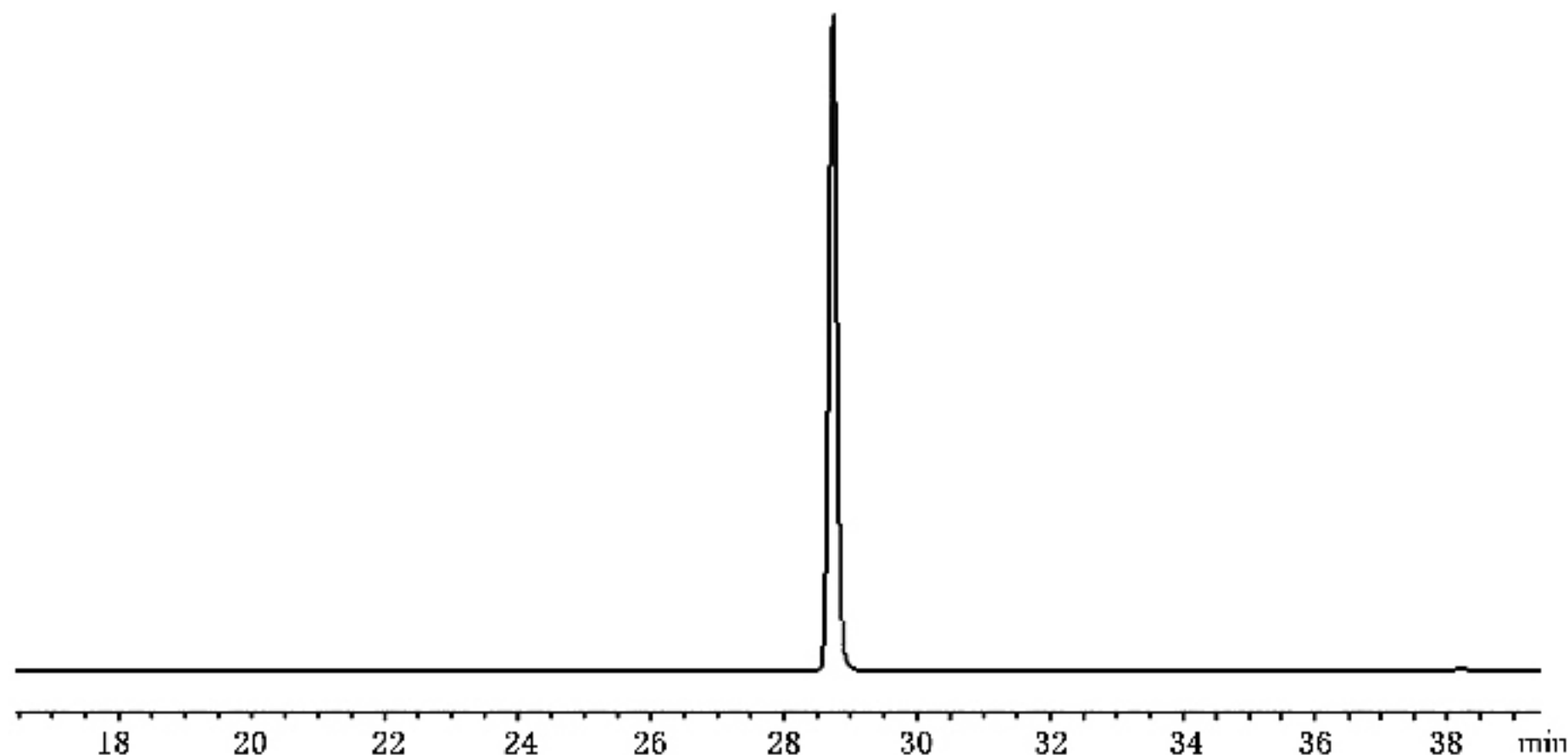
图 E.1 苯并[a]芘参考色谱图
